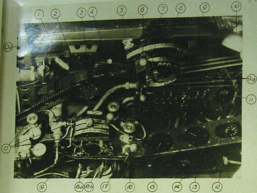
Fig. N° 5. Port Side of Cockpit.
